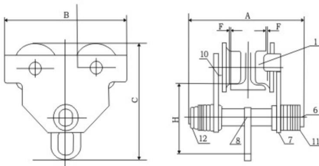
Рисунок 1. Габаритные размеры тележка холостая для тали типа А.
